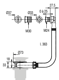
réf. 598300 001 00 tube blanc
