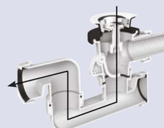
Siphons conçus pour permettre le passage d'un furet (Ø 7 mm). Labellisé solution propre et durable.
