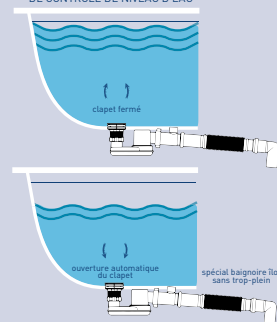
AUTOFLOW : MÉCANISME AUTOMATIQUE DE CONTRÔLE DE NIVEAU D'EAU
