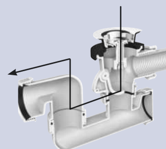
Siphons conçus pour permettre le passage d'un foret (Ø7 mm). Labellisé solution propre et durable.
