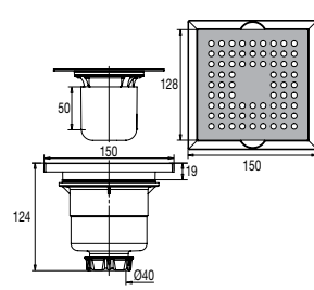
Cadre haute résistance
