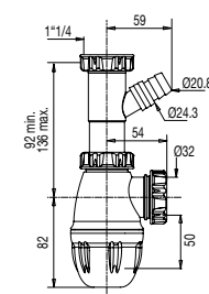
Culot démontable
