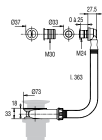
réf. 598300 001 00 tube blanc
