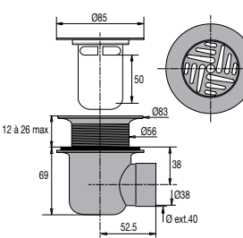
Capot métal et tube garde d'eau
