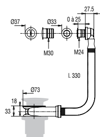
réf. 598300 000 00 tube métallisé
